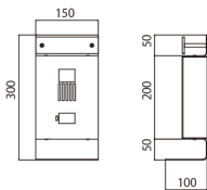
■取付図
