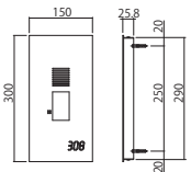
■取付図
