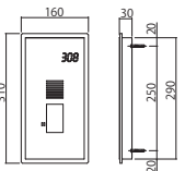
■取付図
